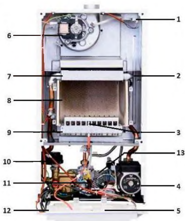
конструкция котла
