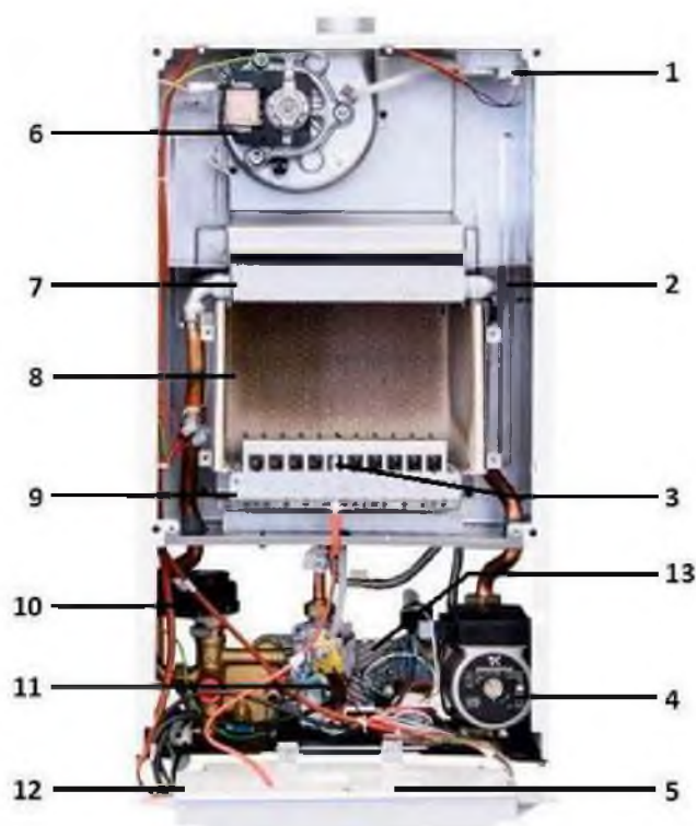
конструкция котла
